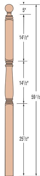
FH4846 3-1/4" Landing Newel
