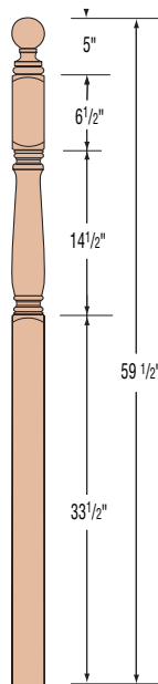
FH4842 3-1/4" Landing Newel
